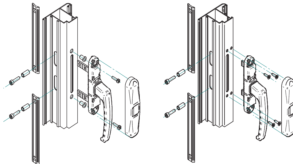
CREMONA IRIA FIJACION APERTURA EXTERIOR CON TUERCAS REMACHABLES DIN 7337
