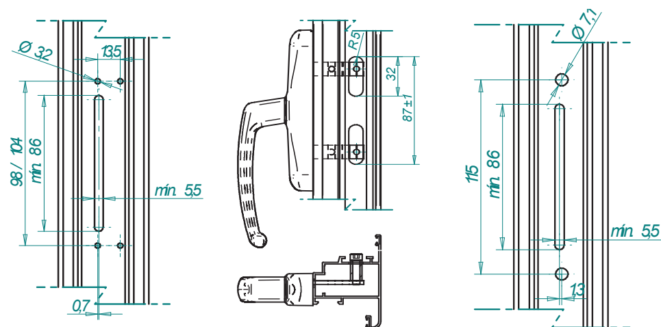
Mecanizado IRIA. DIN 7982 B4,2
