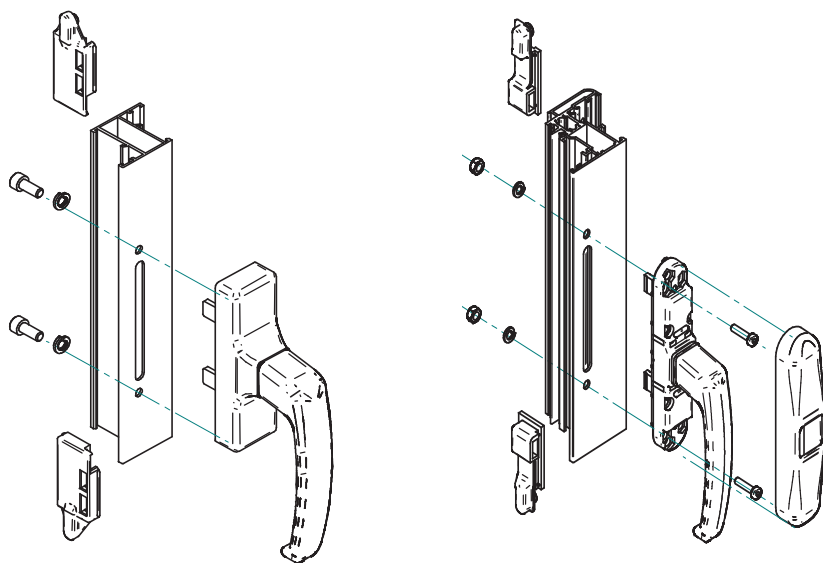
CREMONA FLAVIA FIJACION APERTURA INTERIOR
