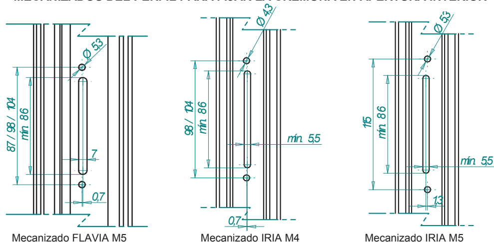
Mecanizado FLAVIA M5
