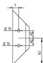
Mecanizados para roseta Mechanising for rosette Usinages pour rosace
