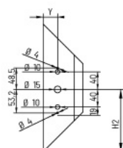
Mecanizados para manilla Mechanising for handles Usinages pour béquille
