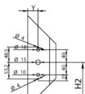
Mecanizados para manilla Mechanising for handles Usinages pour béquille
