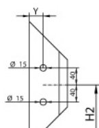
Mecanizados para roseta Mechanising for rosette Usinages pour rosace
