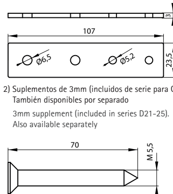
3) Tornillos de 70 mm para perfiles anchos 70 mm screws for thick profiles
